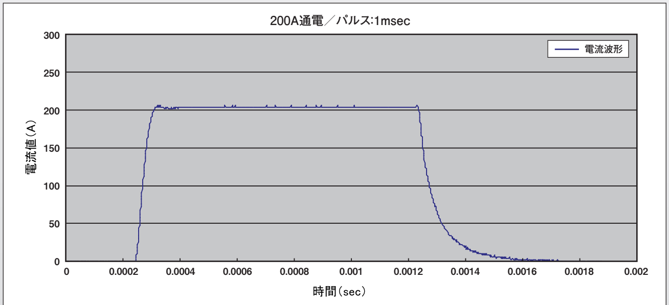
200A 1mS パルス通電波形
